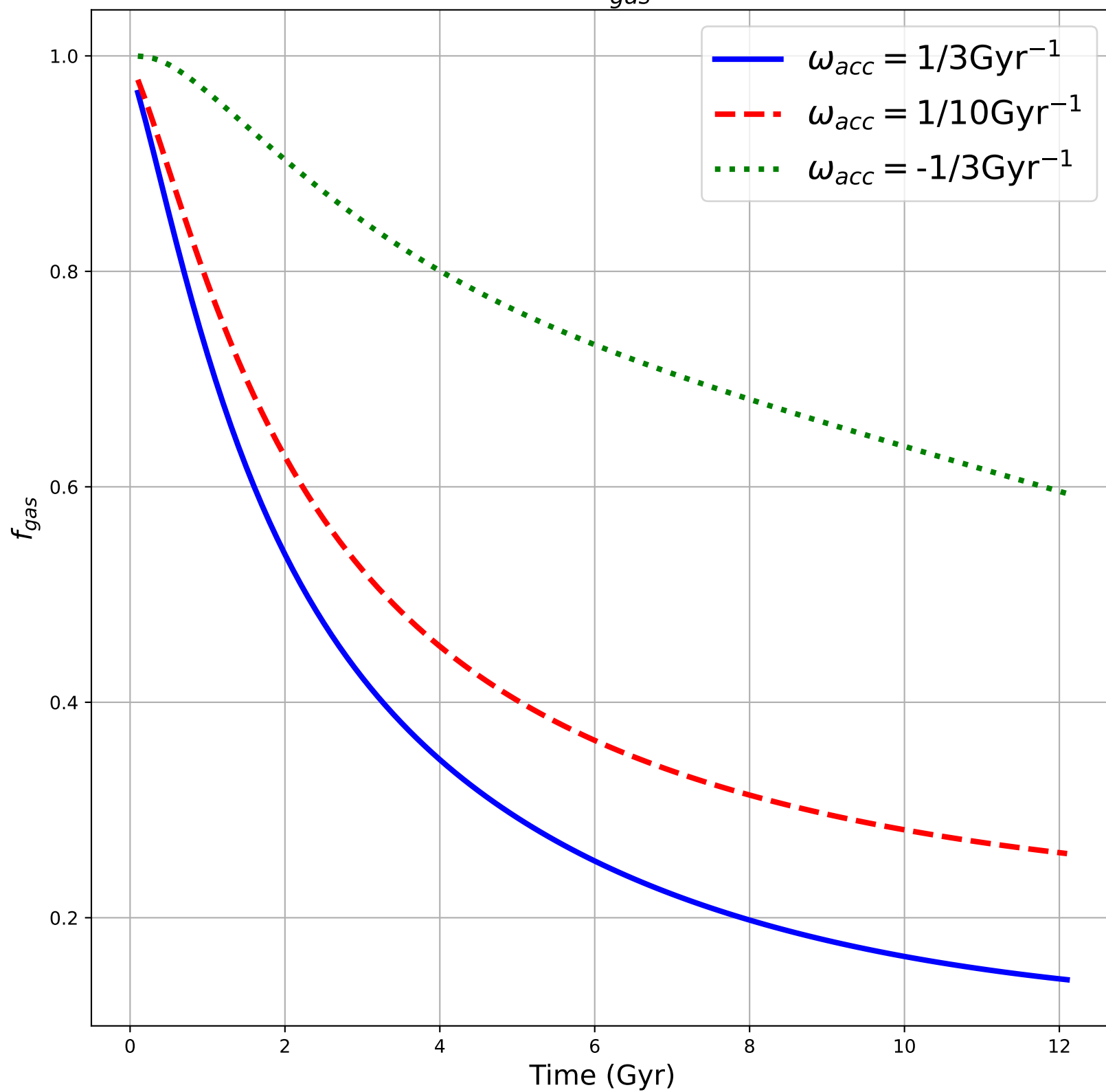
Global f_{gas} vs t
